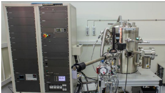
Figura 2: La foto del equipo XPS, PHI 5000 VersaProbe II
