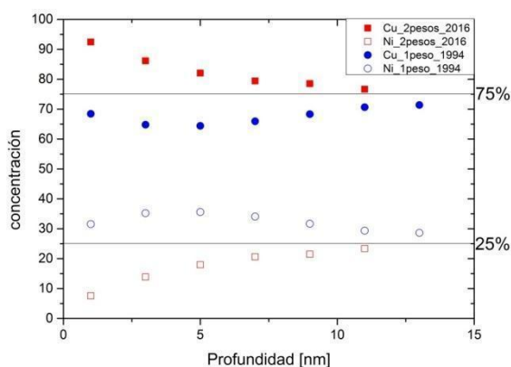
Figura 7: Perfil de profundidad de la parte de plateada de una moneda $1 de 1994 y $2 de 2016, que muestra la evolución de la concentración de Cu/Ni hasta 15 nm de profundidad.
