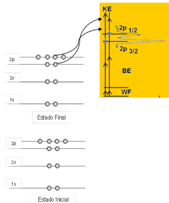
Figura 4: Diagrama del proceso fotoeléctrico
