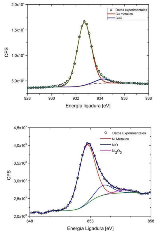
Figura 6: Espectros XPS de alta resolución del Cu 2p_{3/2} y Ni 2p_{3/2} obtenidos en la superficie de la parte del anillo (plateada) de una moneda $1 de Argentina de 1994.
