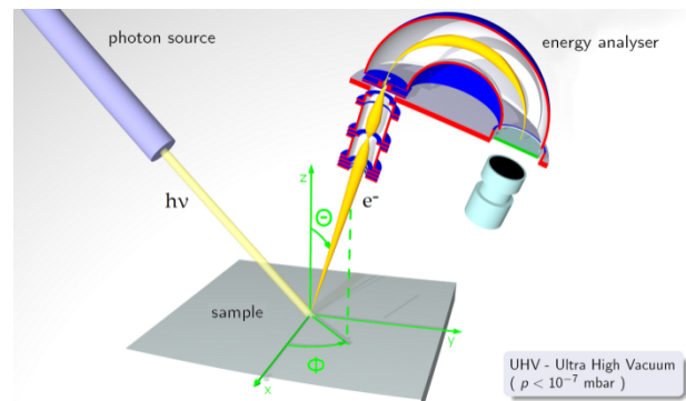
Figura 3: Diagrama de la técnica XPS.
